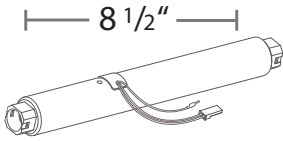
62910-25 RBS Tubular Lithium Motor
